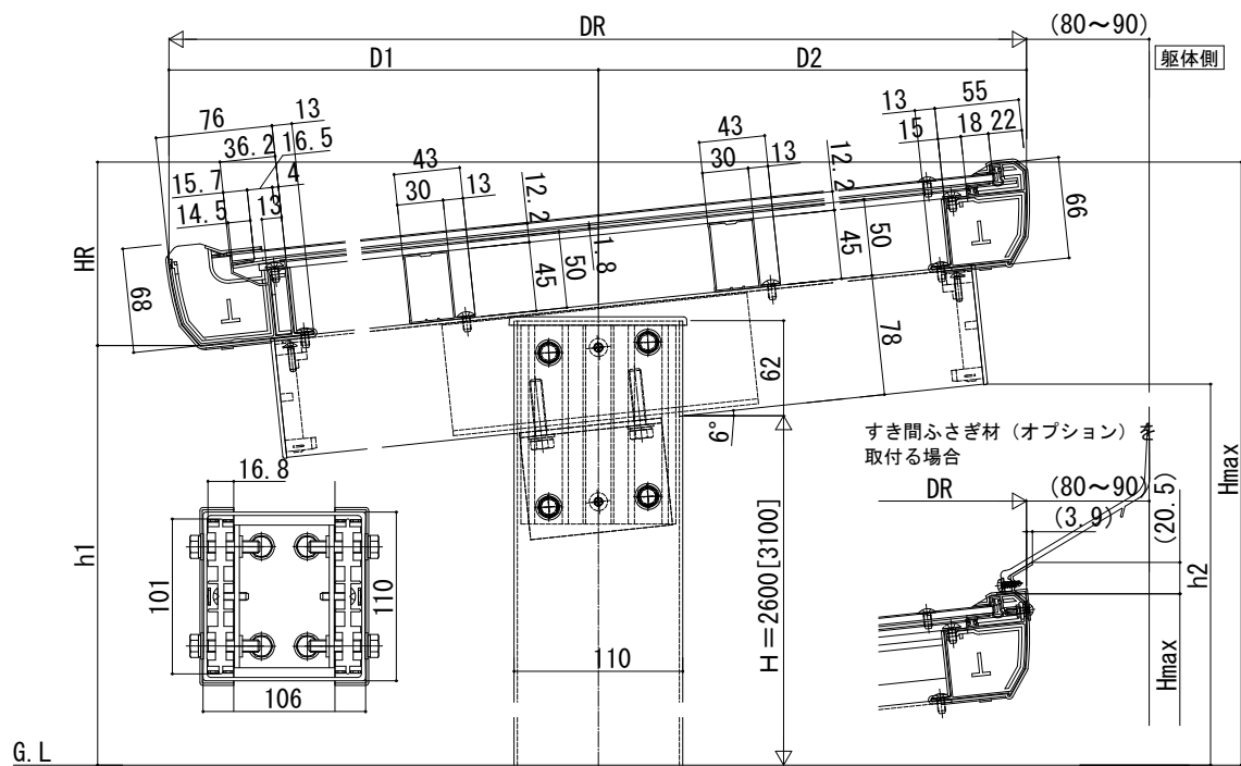
A-A断面
