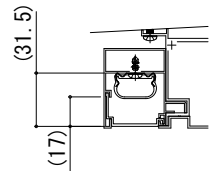
LED照明、照明カバーの納まり図
