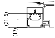
LED照明、照明カバーの納まり図
