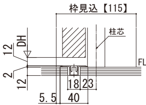
基本寸法表
