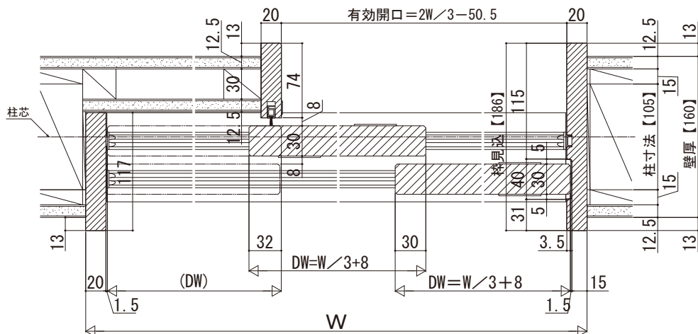
基本寸法表
