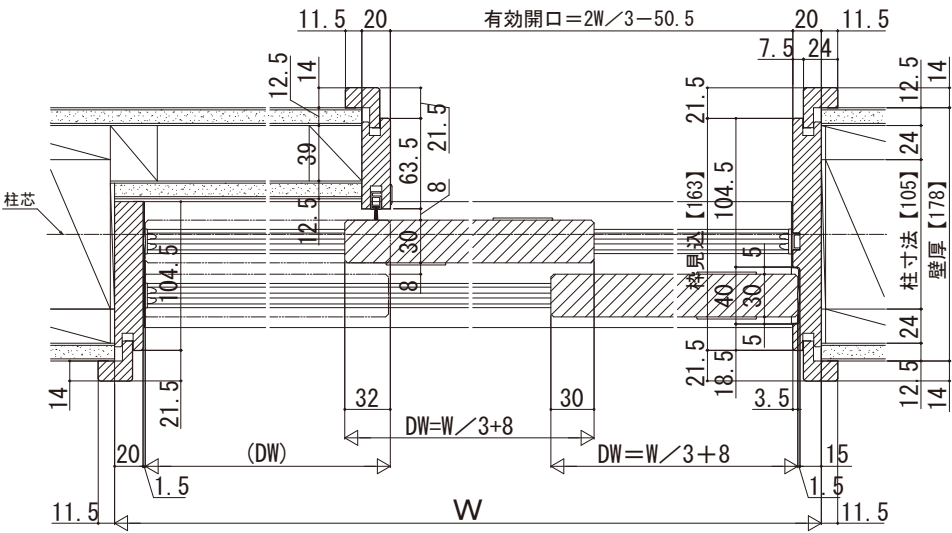
基本寸法表
