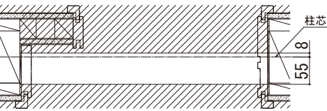
埋込敷居（アルミ）使用時の床貼込み寸法
