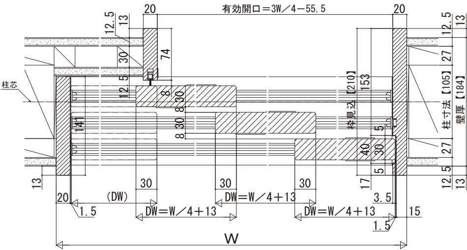
基本寸法表
