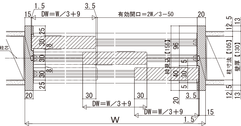
基本寸法表
