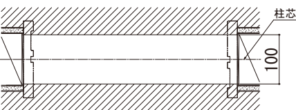
埋込敷居（アルミ）使用時の床貼込み寸法
