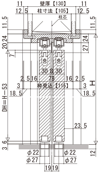
基本寸法表
