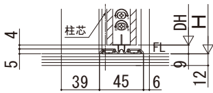
基本寸法表
