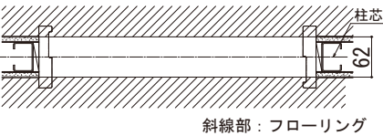
埋込敷居（アルミ）使用時の床貼込み寸法
