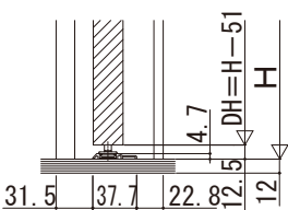
基本寸法表
