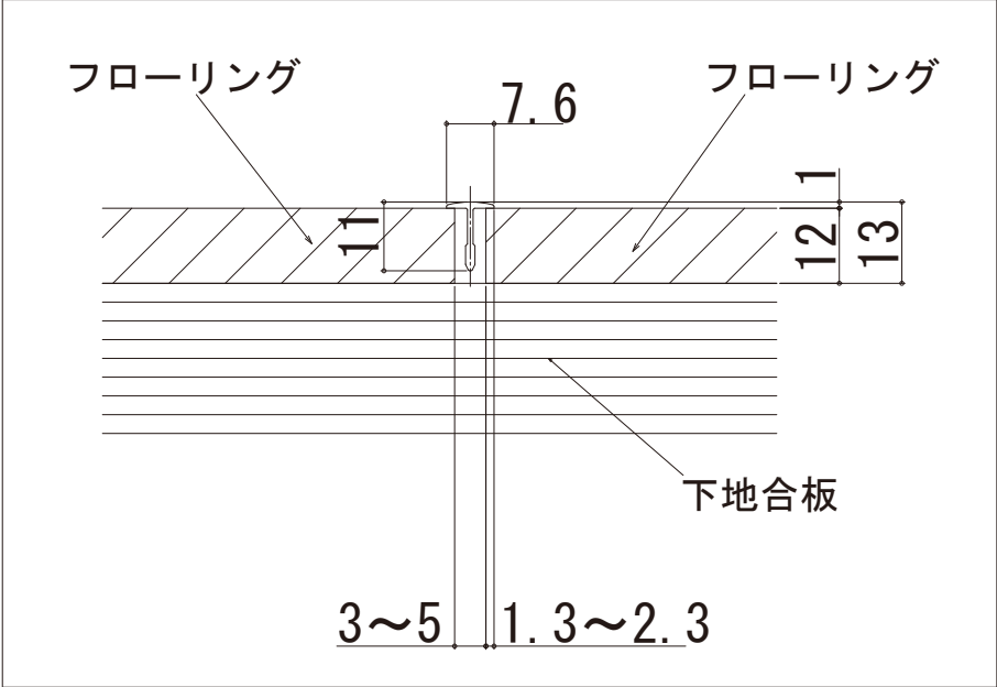
アルミ 詳細図 (2:1)
