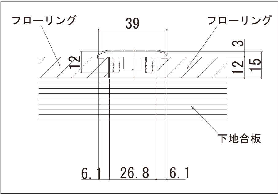
樹脂 詳細図 (2:1)
