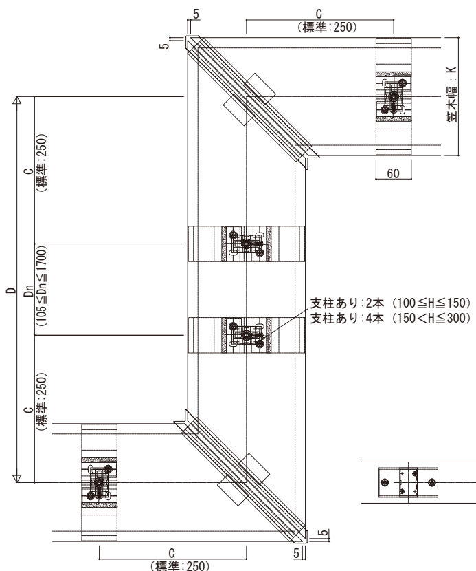
笠木平面図
