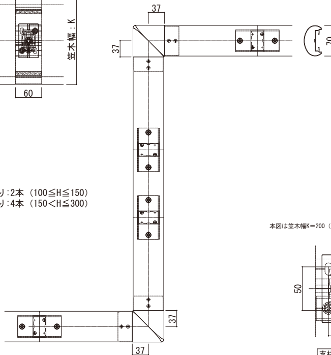
支柱部詳細図
