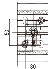
支柱部詳細図
