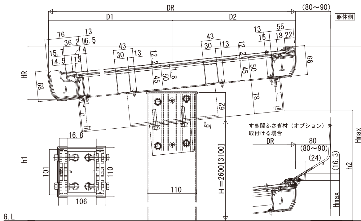
A-A断面
