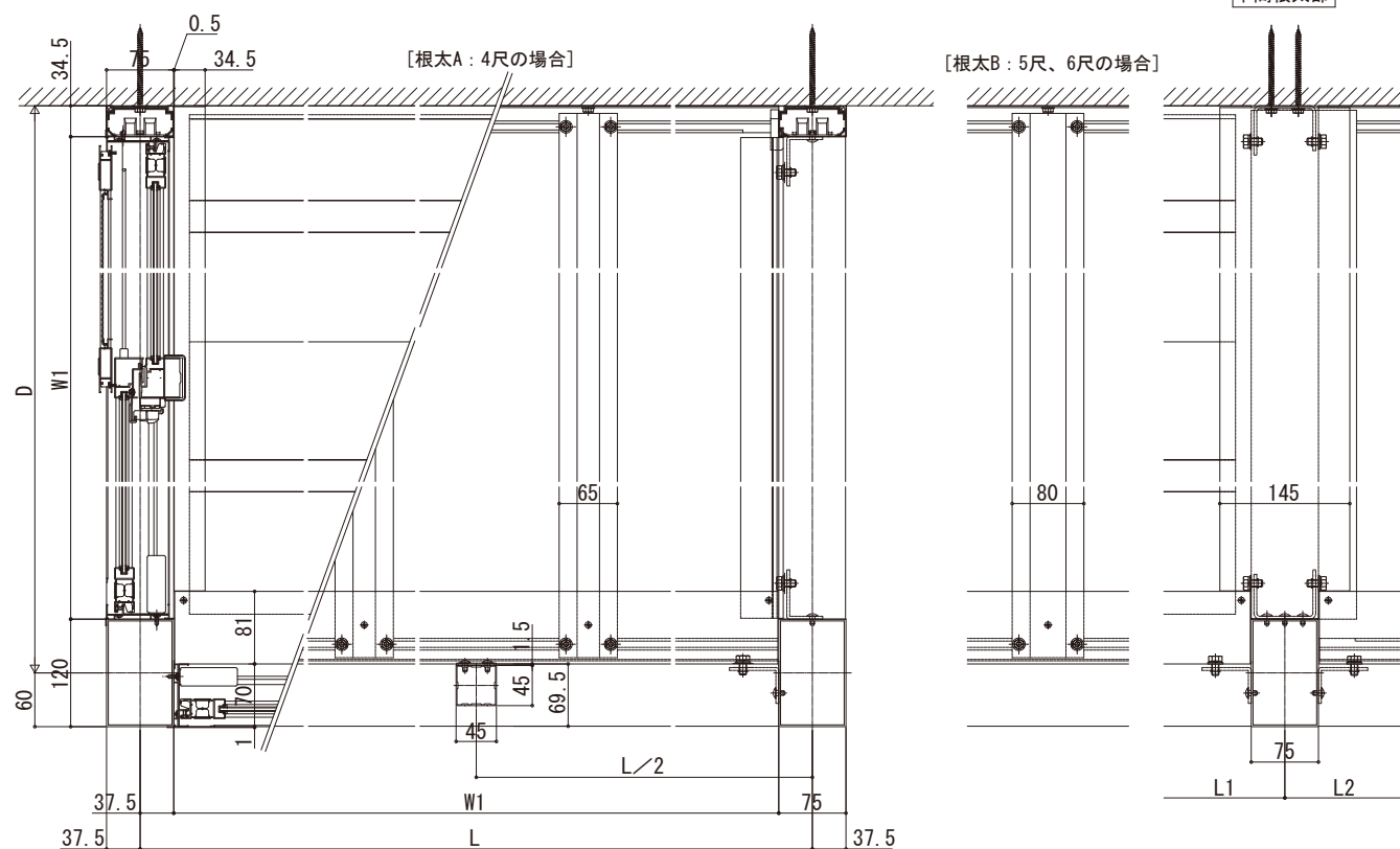
■ジーテラスneo テラス囲い 床納まり
