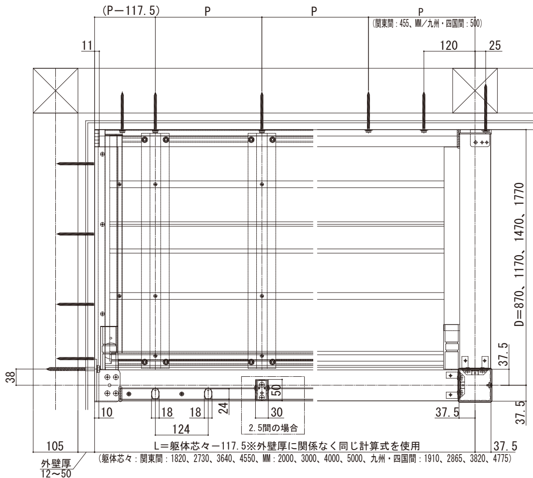
根太掛け補強材部 詳細図
