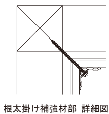
根太掛け補強材部 詳細図
