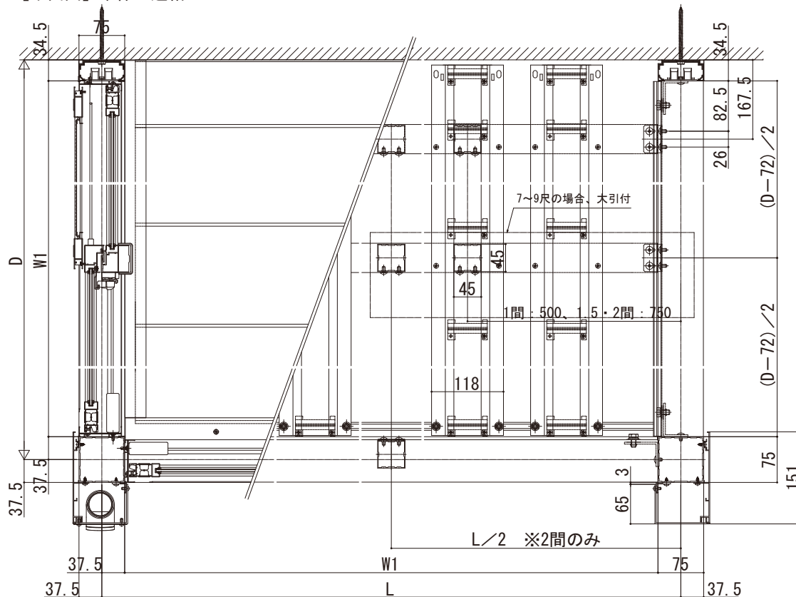
【平面図】単体・連結
