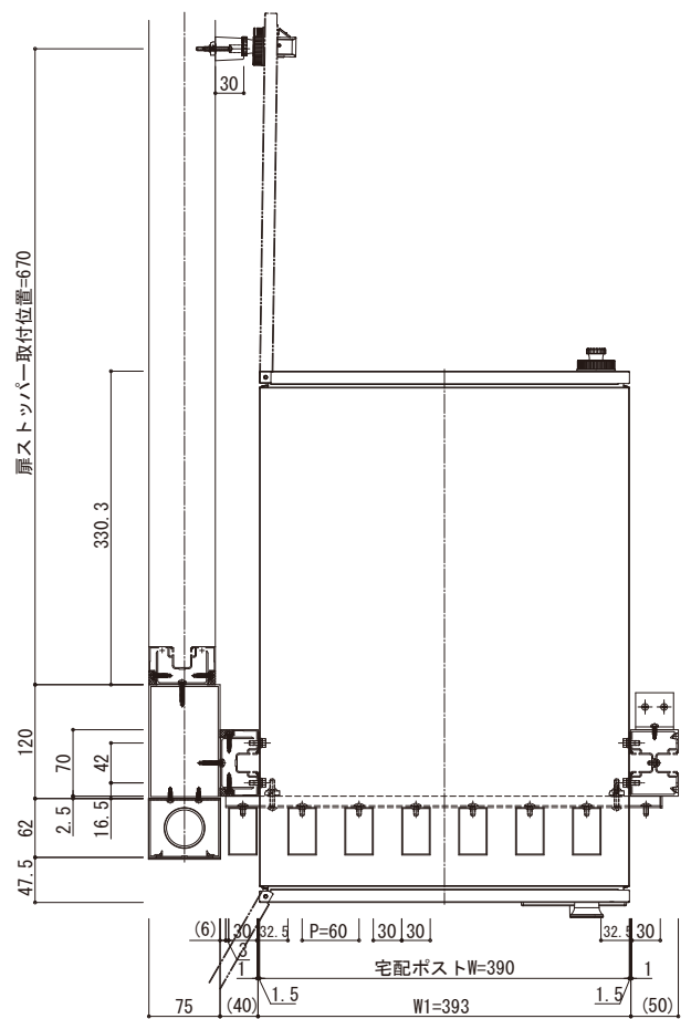
●B-B断面
