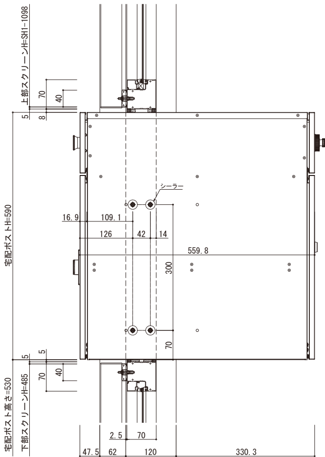
●A-A断面
