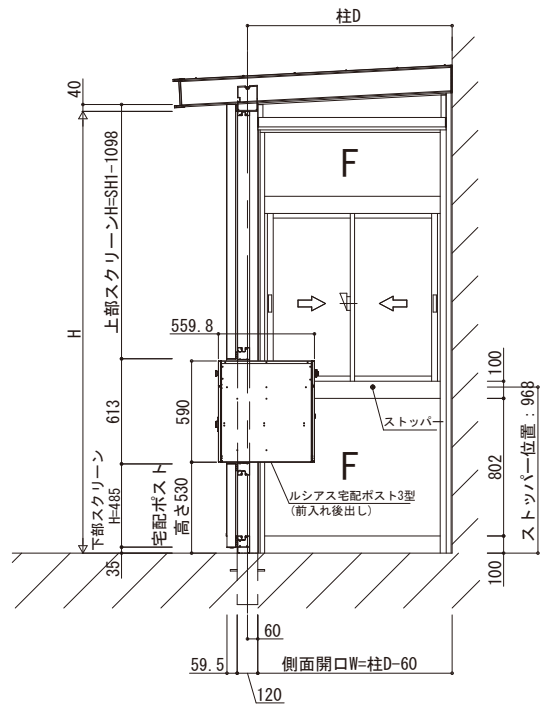
■側面姿図
