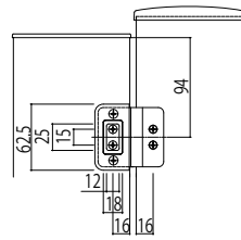
開き防止部品取付部(シンプルオ門扉・ルシアス門扉カテゴリ-Cの場合)
