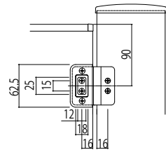
開き防止部品取付部(ルシアス門扉カテゴリ-Bの場合)
