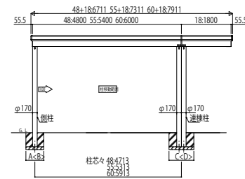
幅延長セット/2台用+α 丸柱 セミハイルーフタイプ・ハイルーフタイプ
