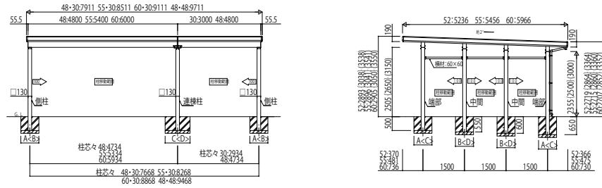
横(2)連棟セット/3台用・4台用 丸柱 標準タイプ
