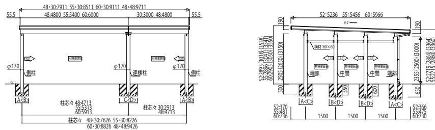
横(2)連棟セット/3台用・4台用 丸柱 セミハイルーフタイプ・ハイルーフタイプ
