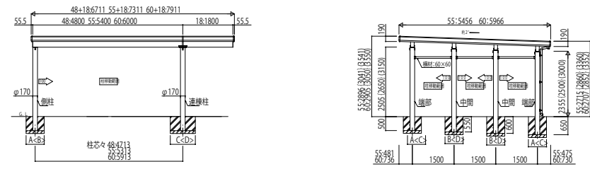
幅延長セット/2台用+α 丸柱 セミハイルーフタイプ・ハイルーフタイプ
