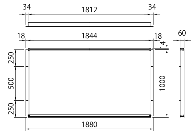
パネル(遮音タイプ H1m) 詳細図 (1/25)
