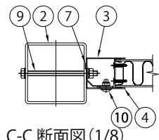
C-C断面図 (1/8)
