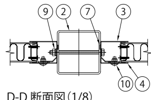
D-D断面図 (1/8)
