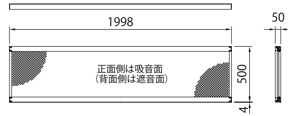
パネル (吸音タイプ H0.5m) 詳細図 (1/25)
