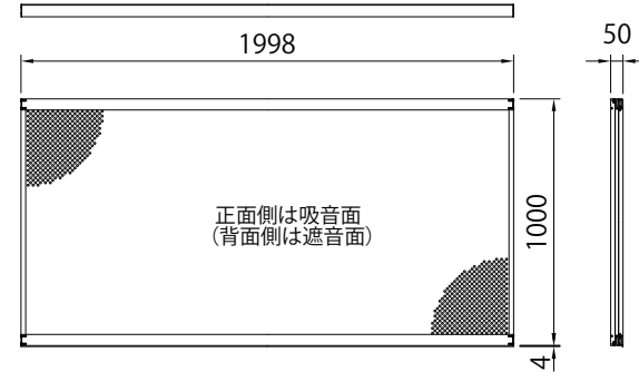
パネル (吸音タイプ H1m) 詳細図 (1/25)
