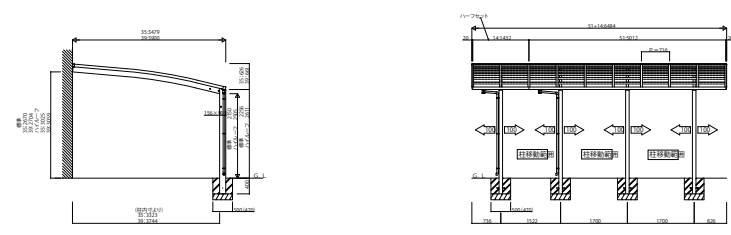
レイナベーカーポート50 サイドパネル
