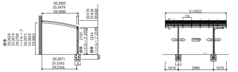
レイナベーカーポート (基本+ハーフ)セット HCA-N
