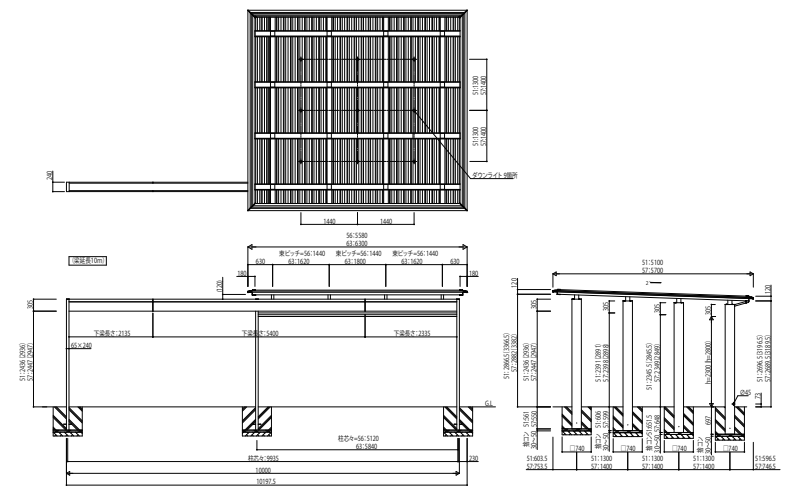
2台用 積雪50cm仕様 梁延長タイプ
