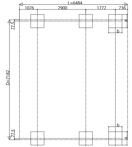
■ 基礎配置図
