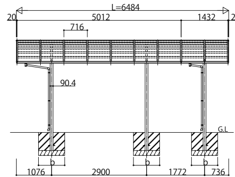
■ 基礎寸法表
