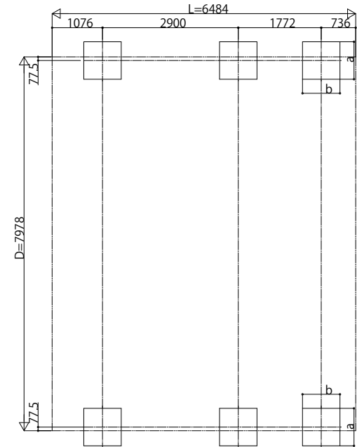
■ 基礎配置図
